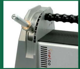
Schleifwinkel-Einstellung von 7,5-90 Grad ergibt einen Spitzwinkel zwischen 15 und 180 Grad.
